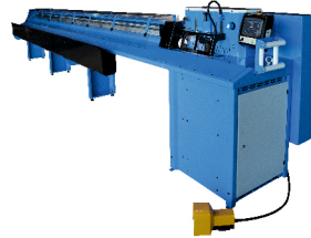
CM 75 QT Yarı Otomatik Hortum Kesme Makinası 2"e kadar R1-R2-4SH hortumları keser 6 Metre kesme tablası +Ayak pedalı +Duman atıcı Bilgisayar kontrol özelliği vardır
